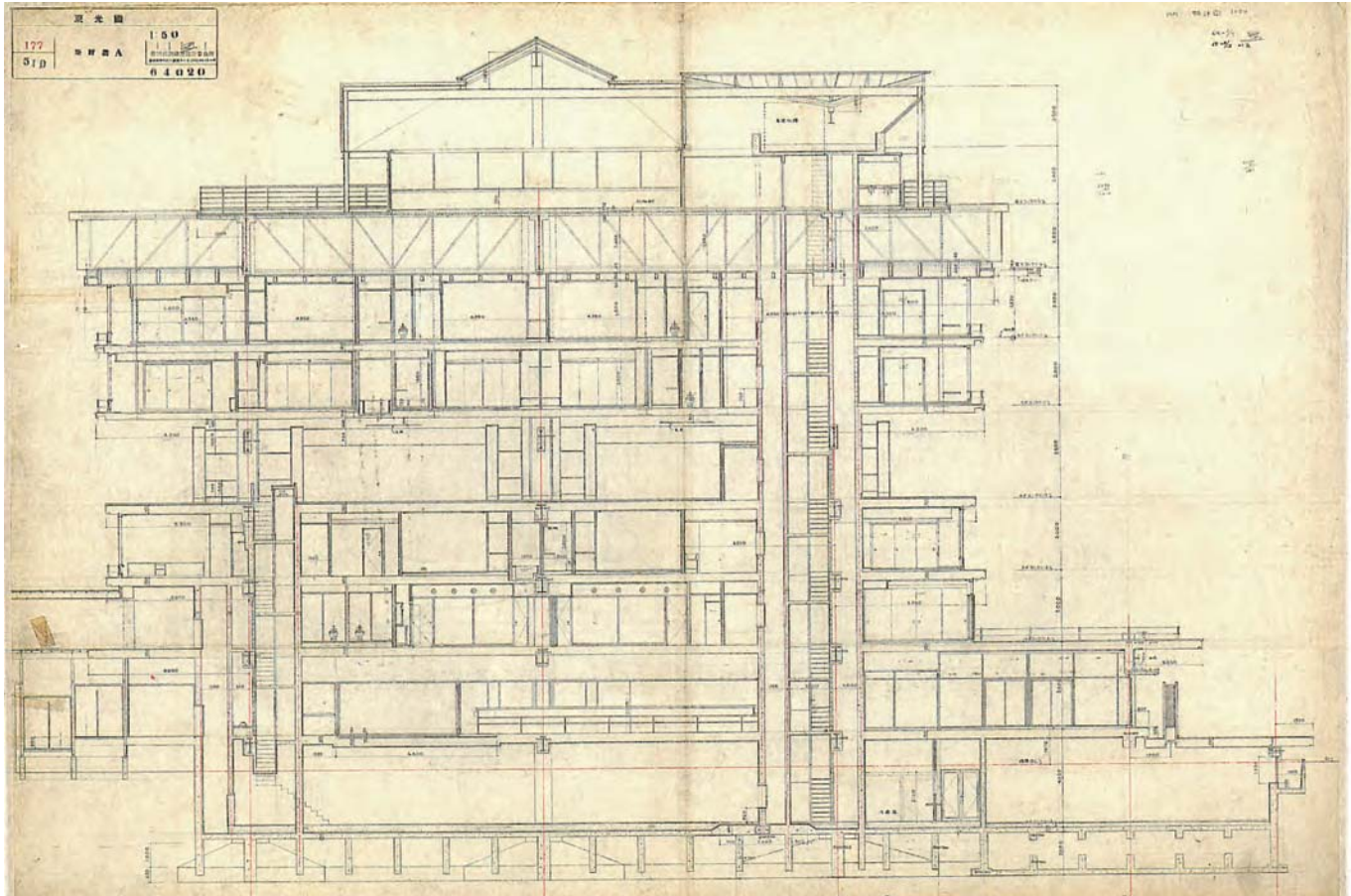
図面提供：情報建築・スミス睦子・菊竹雪・大上かすみ・菊竹三訓
